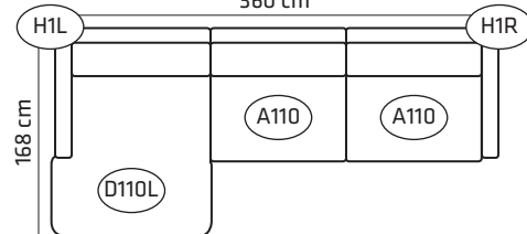
H1L-D110L-A110-A110-H1R
